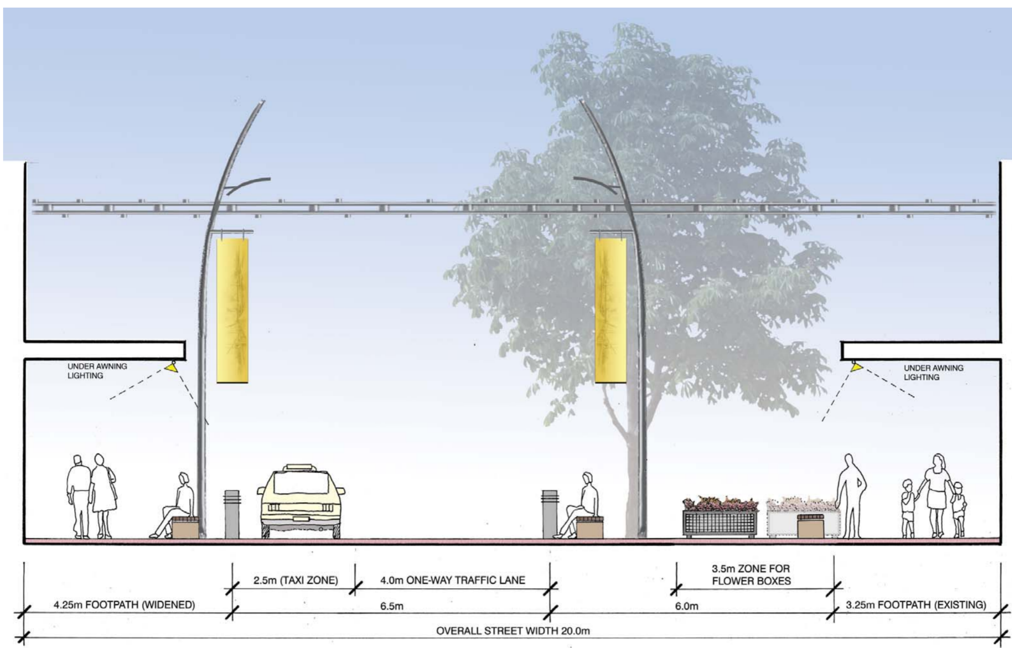
Section A-A
